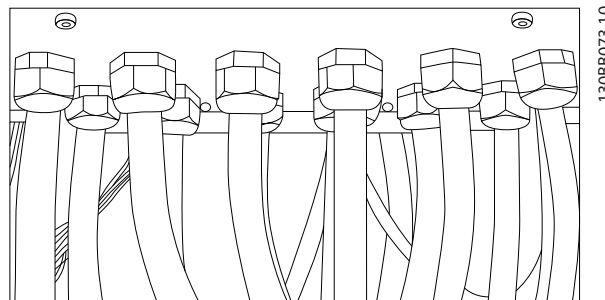
Рисунок 3.23 Пример правильной установки панели уплотнений
